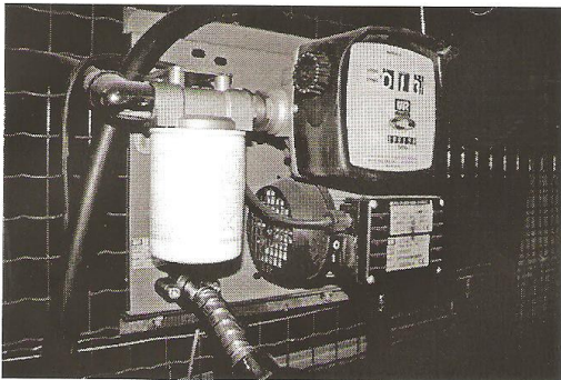
Débitmètre gasoil de l'atelier communal.
